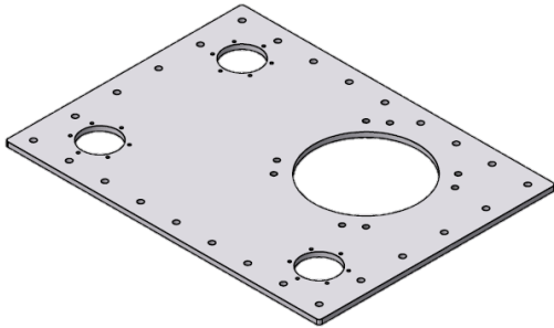
Lokk for cyclonetank 60/120 liter Tegn. nr. 305-009-P02 Art.nr: 305009P02
